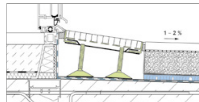
Durch den rampenartig einstellbaren Drainrost AquaDrain® BF-FLEX liegt die Oberkante der am Türelement angeflanschten Abdichtung nicht mehr unter der Oberkante des Belages. Die rückstaufreie Entwässerung erfolgt in die AquaDrain® Hochleistungsdrainagen.
