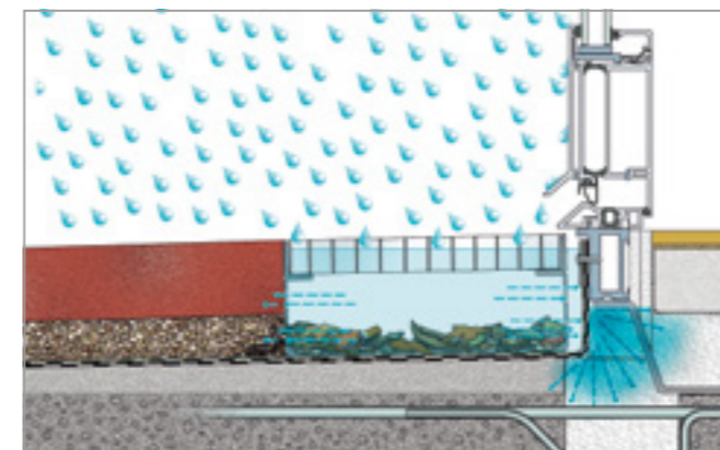
Bei Drainrosten ohne Schmutzgitter kann die Entwässerungsleistung durch hereinfallenden Schmutz erheblich beeinträchtigt werden. Ein Rückstau führt zu hinterläufigem Wasser mit Feuchteschaden.
