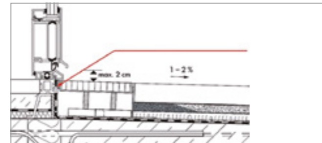
Kritischer Anschlusspunkt: Die oberste Befestigung der Abdichtung liegt unter der Oberkante des Belages.
